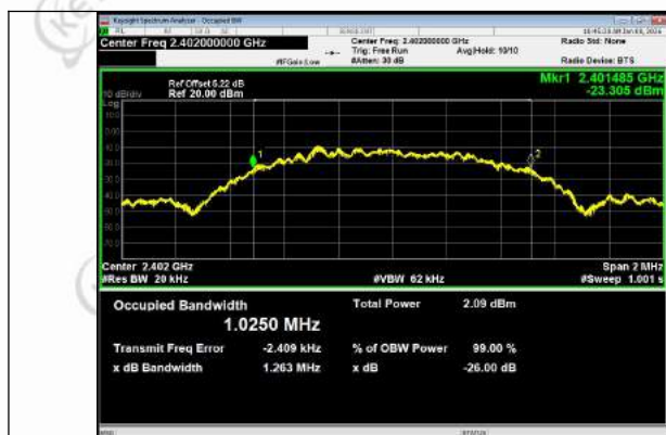
BLE 1M_Channel 0
