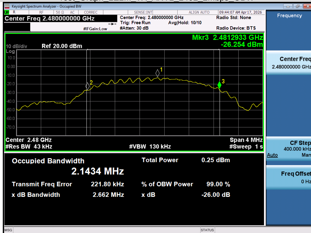
Test_Graph_LE2M_TX_ANT1_2480_2Mbps_OBW
