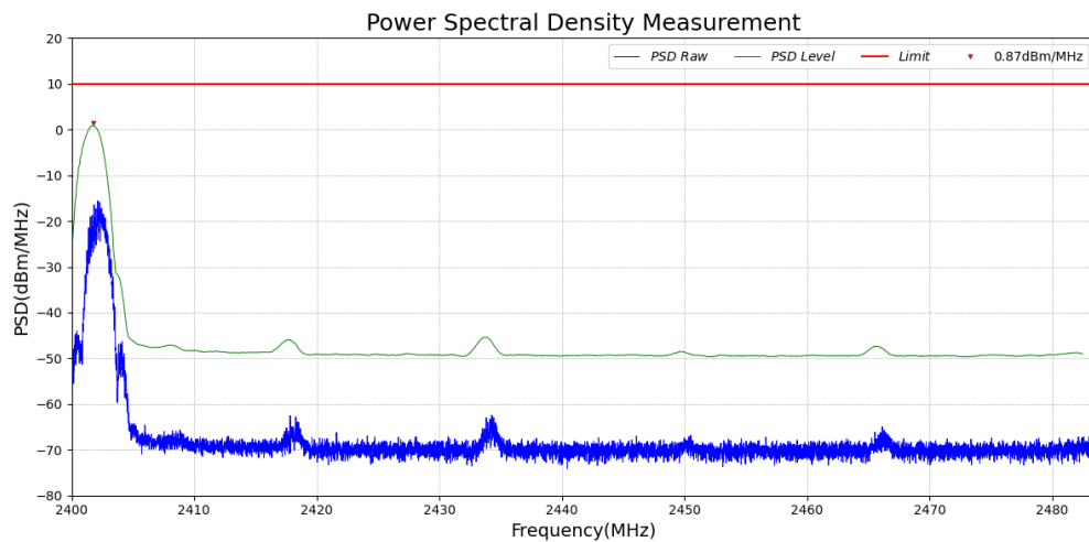
Test_Graph_LE2M_TX_ANT1_2402_2Mbps_PSD
