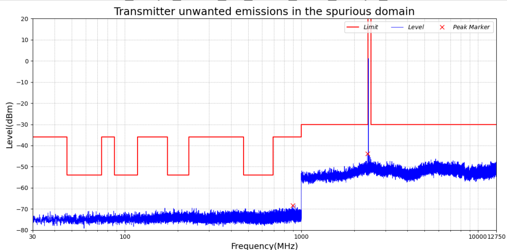
Test_Graph_LE2M_TX_ANT1_2402_2Mbps_TX
