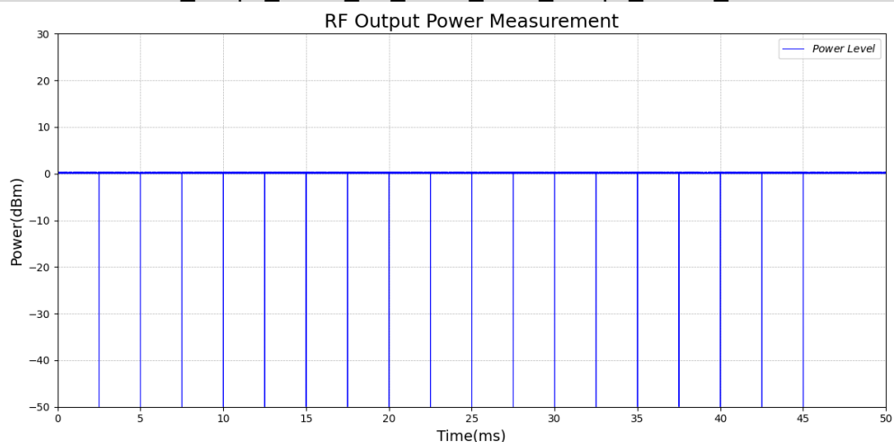
Test_Graph_LE2M_TX_ANT1_2480_2Mbps_Power_NT
