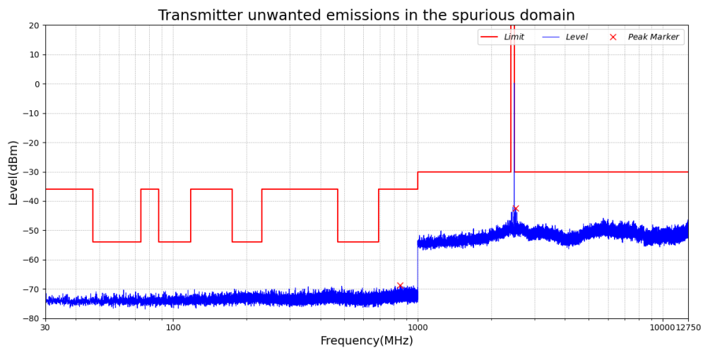
Test_Graph_LE1M_TX_ANT1_2480_1Mbps_TX
