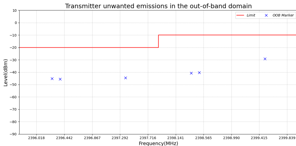
Test_Graph_LE2M_TX_ANT1_2402_2Mbps_OOB_L
