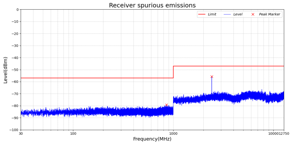
Test_Graph_LE2M_RX_ANT1_2480_2Mbps_RX
