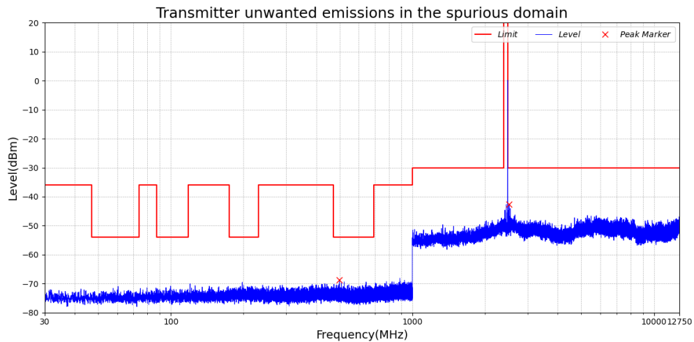
Test_Graph_LE2M_TX_ANT1_2480_2Mbps_TX
