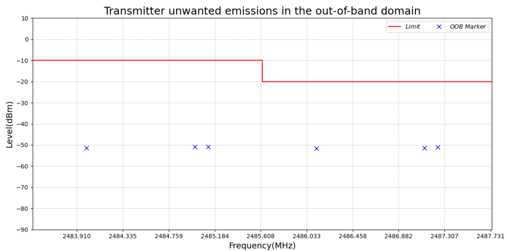
Test_Graph_LE2M_TX_ANT1_2402_2Mbps_OOB_R
