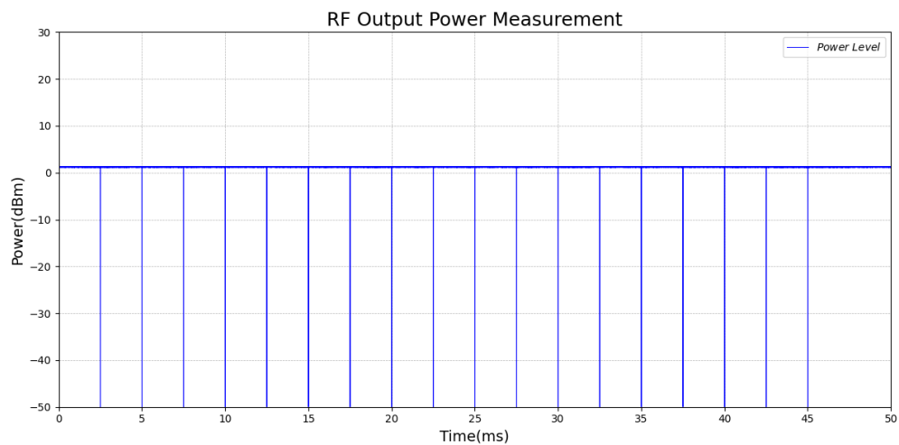
Test_Graph_LE2M_TX_ANT1_2402_2Mbps_Power_NT
