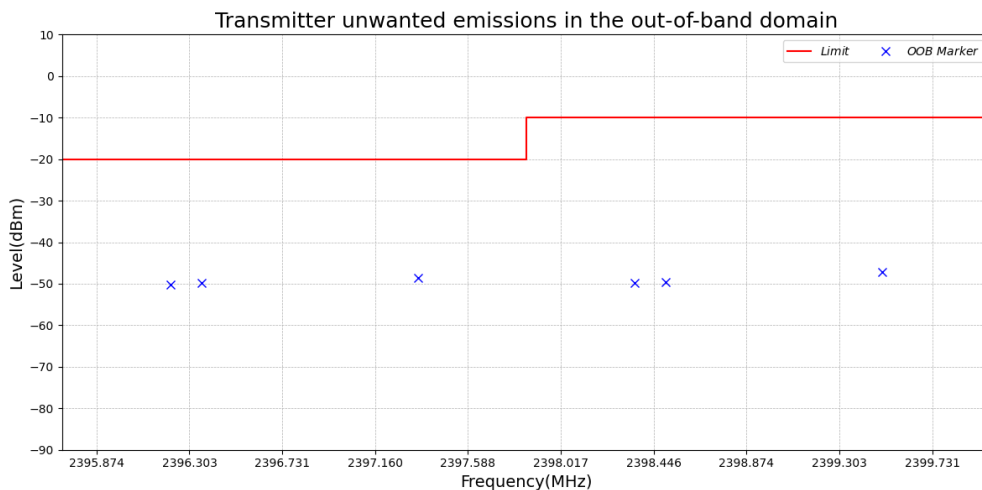
Test_Graph_LE2M_TX_ANT1_2480_2Mbps_OOB_L
