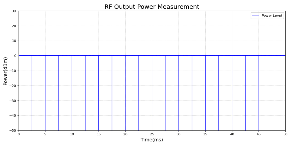
Test_Graph_LE2M_TX_ANT1_2480_2Mbps_Power_HT
