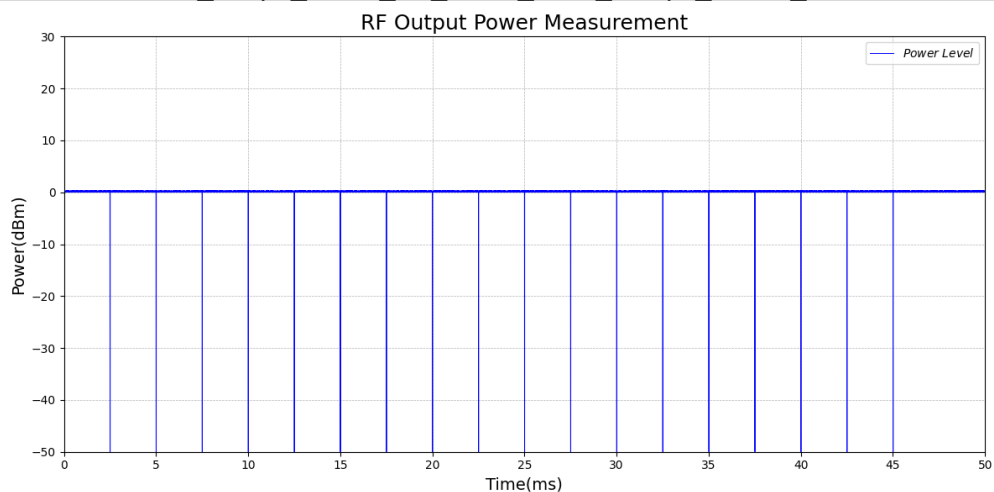
Test_Graph_LE2M_TX_ANT1_2480_2Mbps_Power_LT
