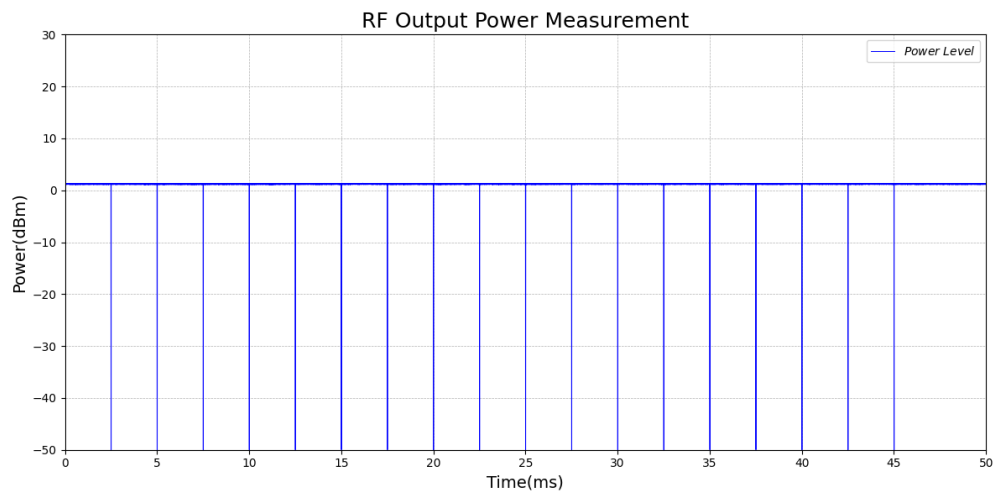
Test_Graph_LE2M_TX_ANT1_2402_2Mbps_Power_LT
