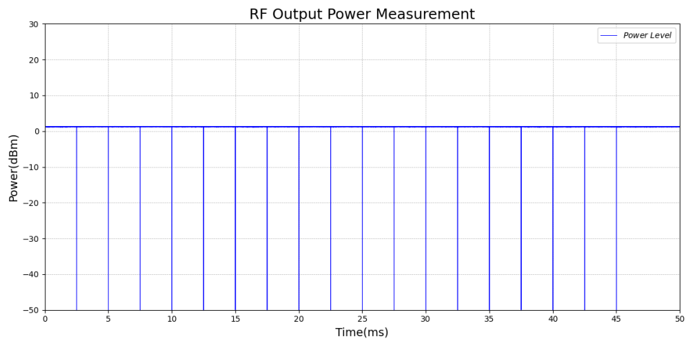
Test_Graph_LE2M_TX_ANT1_2402_2Mbps_Power_HT
