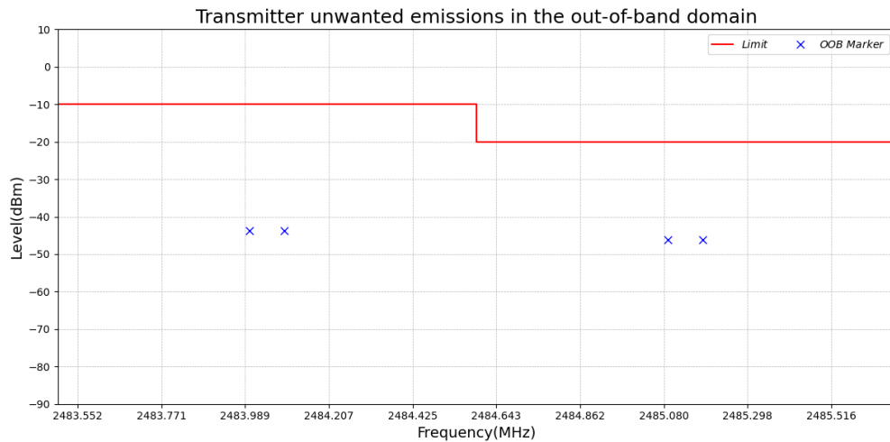
Test_Graph_LE1M_TX_ANT1_2480_1Mbps_OOB_R
