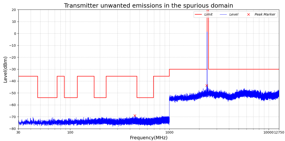
Test_Graph_LE1M_TX_ANT1_2402_1Mbps_TX
