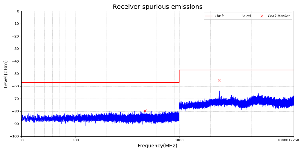
Test_Graph_LE2M_RX_ANT1_2402_2Mbps_RX
